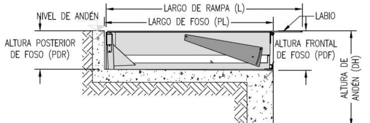
Vista Lateral
