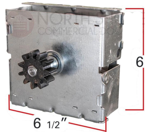
MECANISMO DE 6 1/2" DE ANCHO POR 6" DE ALTO POR 2 1/2" DE FONDO.
