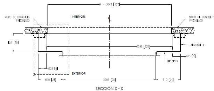
SECCIÓN X - X
